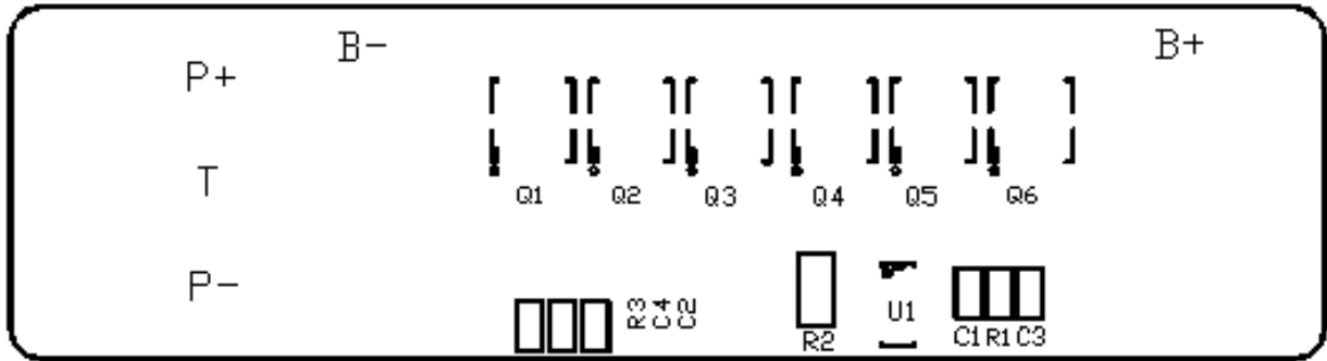
TopOverlay
